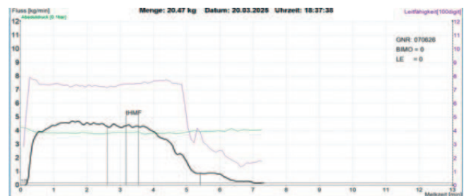
Aufgezeichnete Milchflusskurve eines Lactocorders
